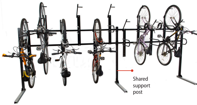
MaxRack Stand w/Modular Add-on Unit
